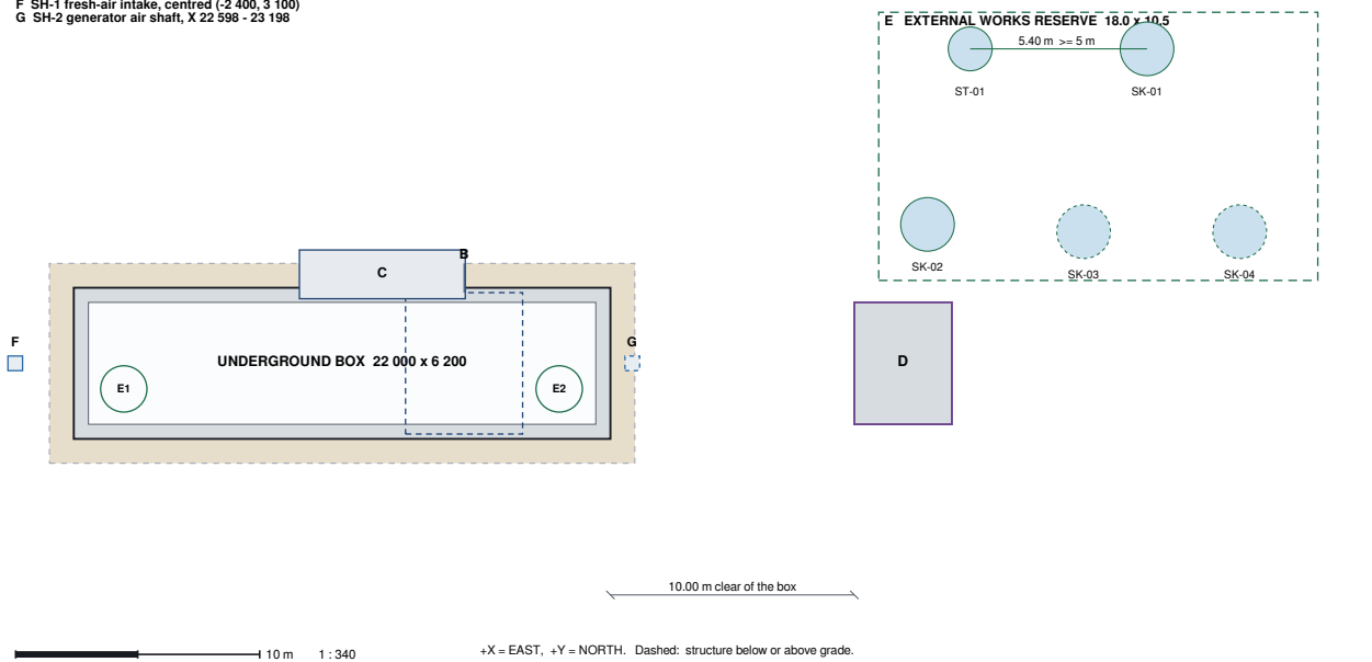
Fig 2.1 : Site Layout Plan
