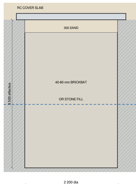
SK-01 / SK-02 SOAK PIT 1 : 55
